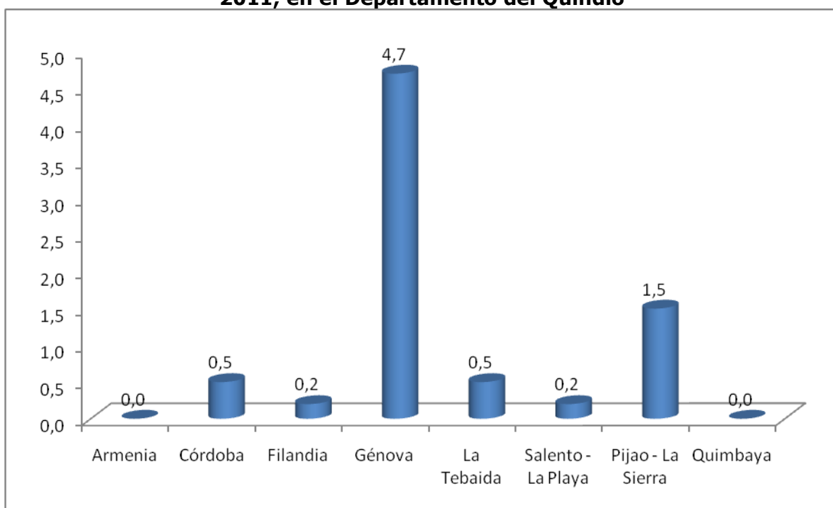
Grafica 1. Precipitación registrada a las 7:00 am el día 02 de Diciembre de 2011, en el Departamento del Quindío
